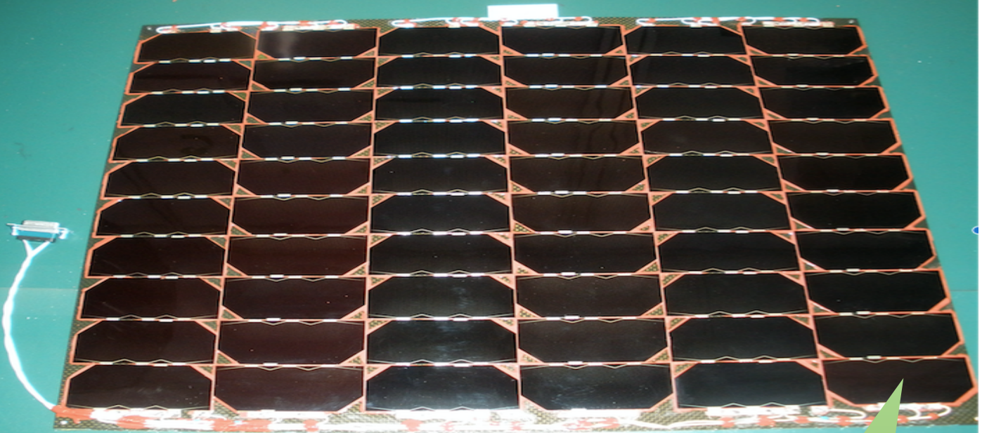
写真：PROCYON搭載太陽電池パネル (20直列、3並列 サイズ487 x440)
